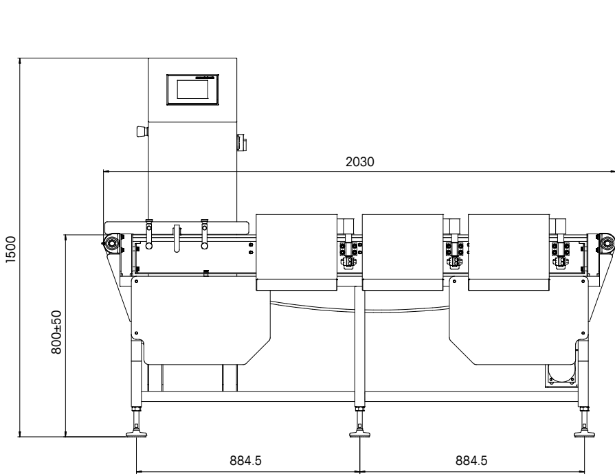
XG 300/6 分选机示意图 - 典型尺寸 (单位: mm)
