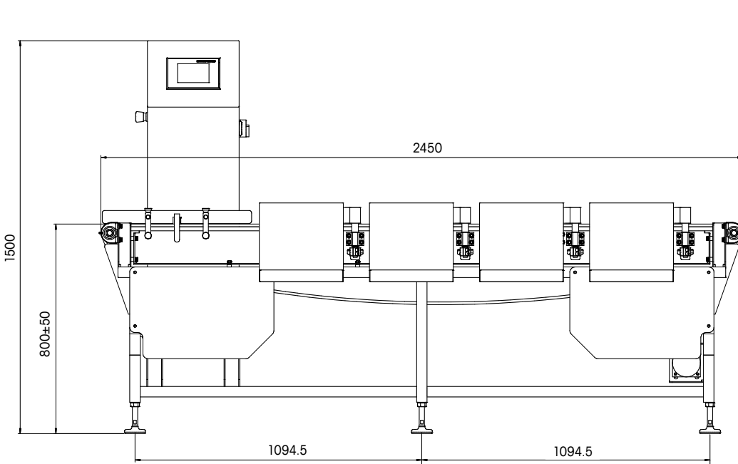
XG 300/8 分选机示意图 - 典型尺寸 (单位: mm)
