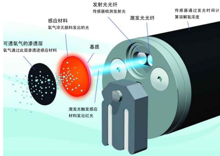
图1. 传感器发射蓝光, 从而引发感应材料产生红光。产生的红光因氧气的存在而发生变化, 传感器测量到的变化与溶解氧浓度成正比。比较蓝光触发的红光信号与参比的红光信号(图2), 然后计算出一个稳定的溶解氧浓度。
