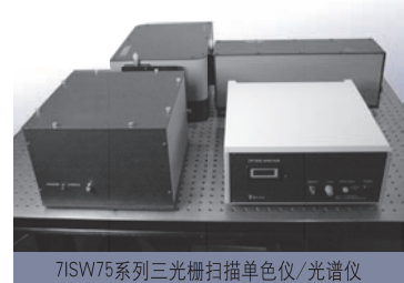
7ISW75系列三光栅扫描单色仪/光谱仪
