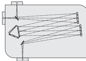
光路图
