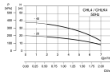
水泵性能曲线 / Performance curve
