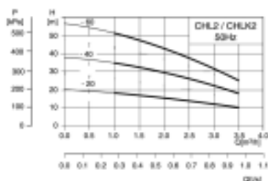
水泵性能曲线 / Performance curve
