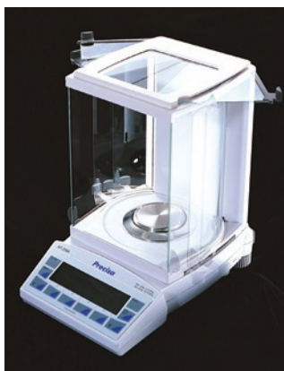
抗靜電玻璃防風罩，採用三門雙向開啓， 隱藏式設計節省置放空間、安全可靠
