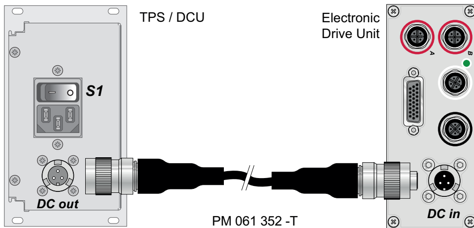
图片 18： 将电子驱动装置连接到电源包
