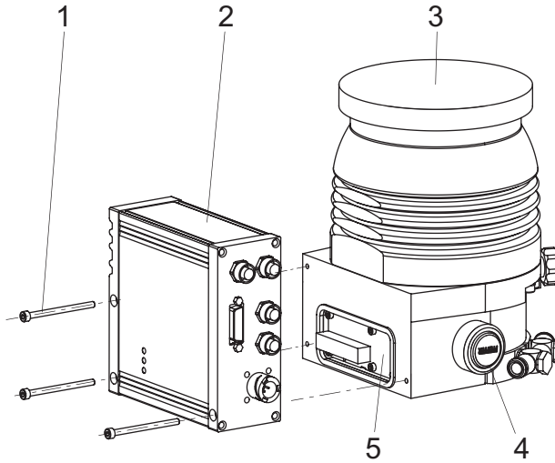
图片 22: 电子驱动单元 TC 400 的安装
