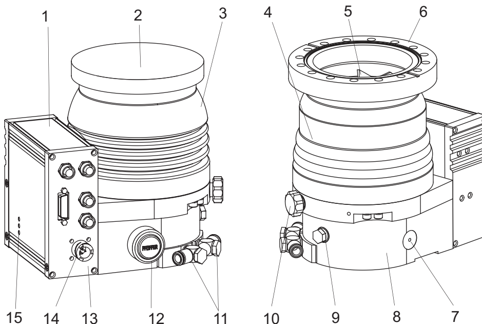
图片 3: HiPace 300 设计
