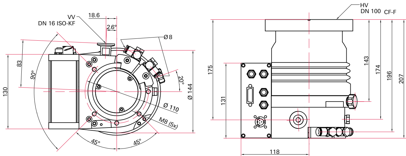
图片 25: HiPace 300 | TC 400 | DN 100 ISO-F 尺寸
