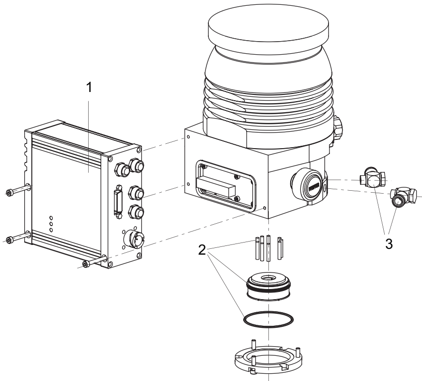
图片 23: HiPace 300 的备用件
