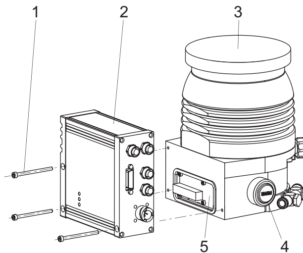
图片 21： 电子驱动单元 TC 400 的拆卸
