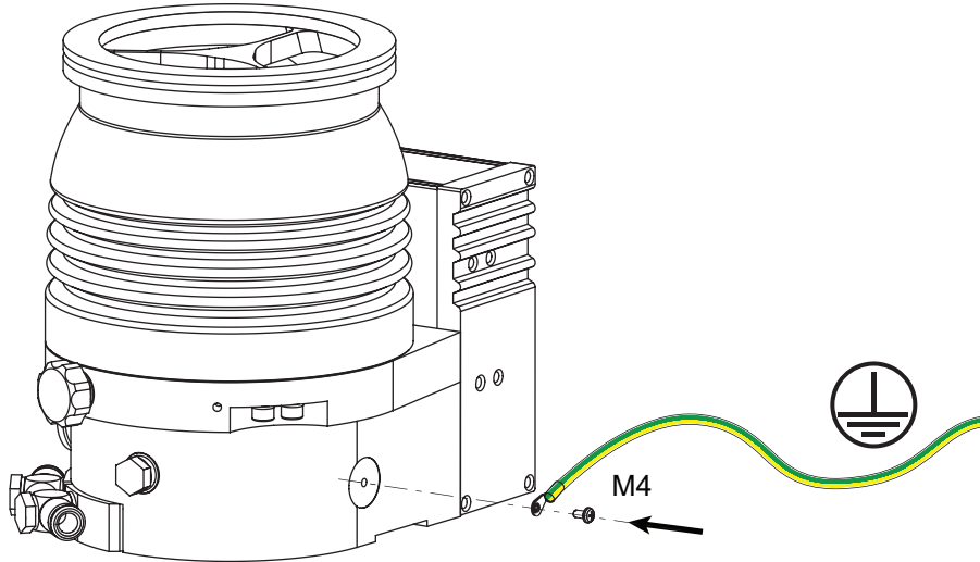
图片 17： 示例:连接接地电缆
