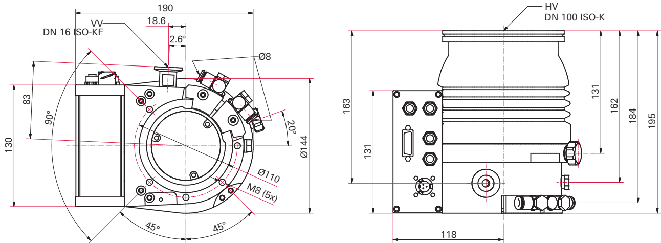
图片 24: HiPace 300 | TC 400 | DN 100 ISO-K 尺寸
