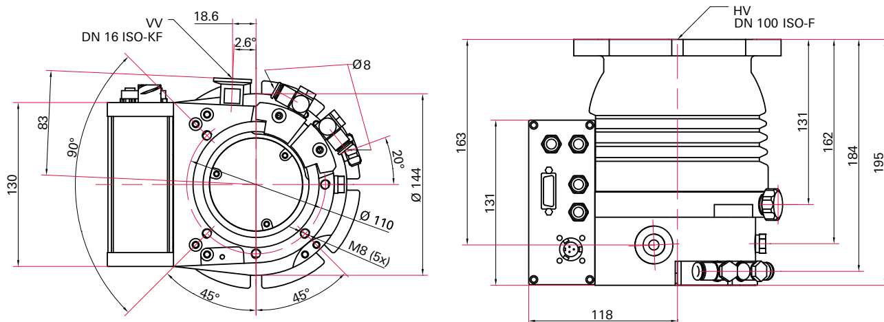
图片 26: HiPace 300 | TC 400 | DN 100 CF-F 尺寸
