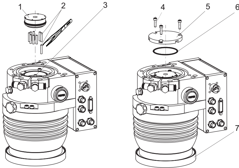
图片 20: 安装油绵
