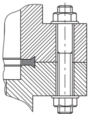
图片 15: CF-F 法兰连接, 螺杆和通孔
