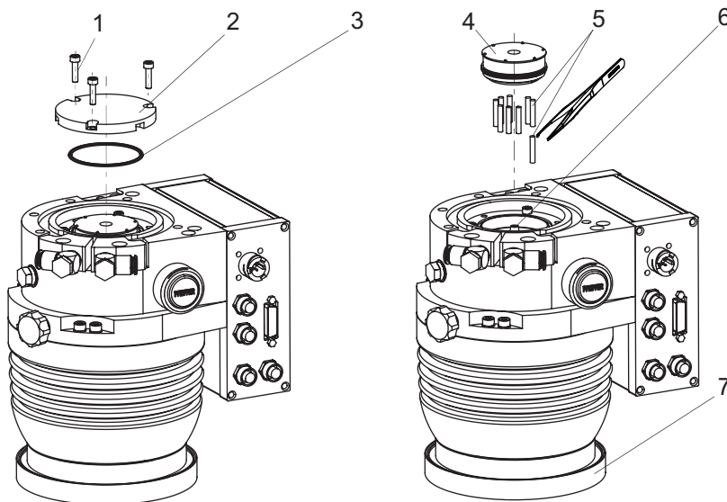
图片 19: 拆下油绵
