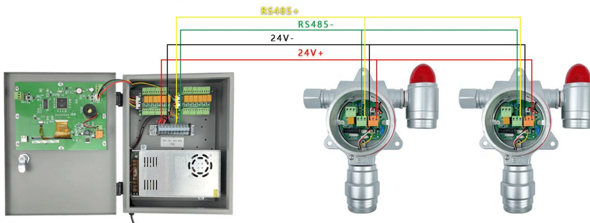
主机与检测仪RS485接线示意图
