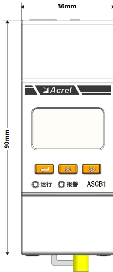
图3 智能网关外形尺寸图
