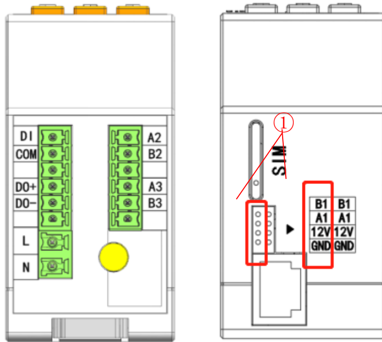
图 4 智能网关接线端子示意图
