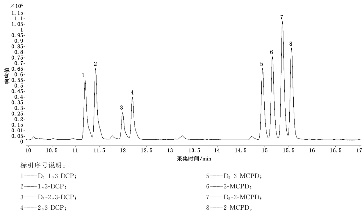
图 A.1 标准溶液(0.10 μg/mL)中氯丙醇及其同位素内标衍生物的色谱图
