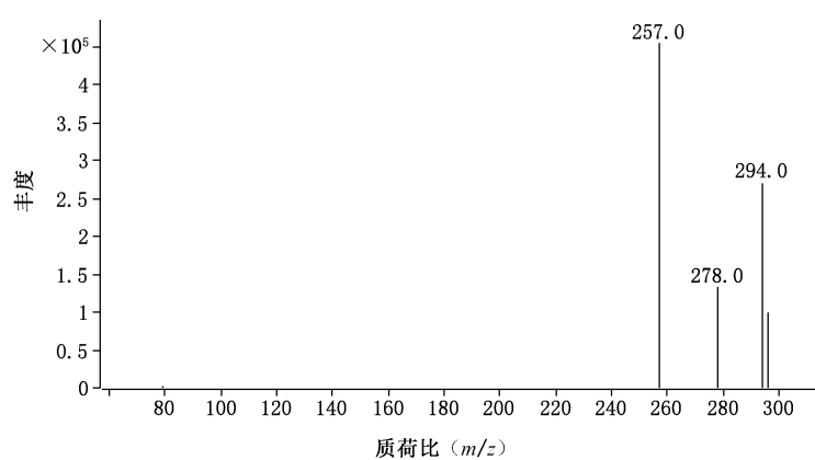
e) D_5 -3-MCPD
