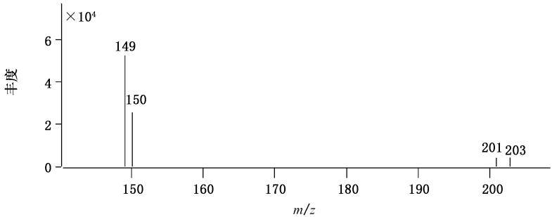
b) D_5 -3-MCPDE
