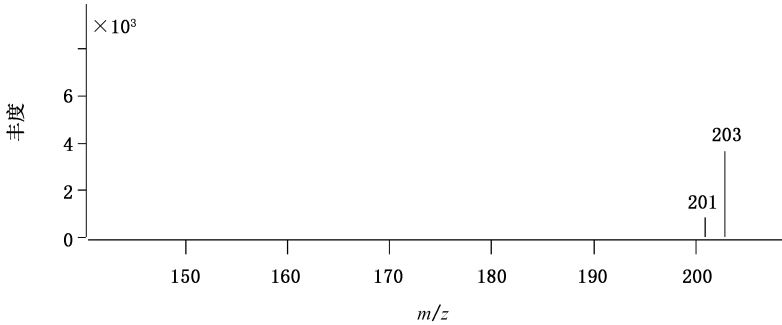
d) D_5 -2-MCPDE
