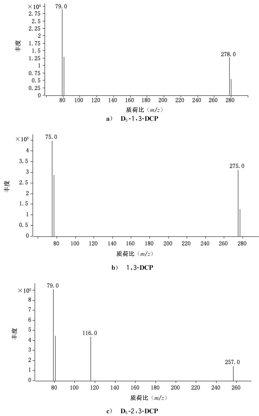
图 A.2 标准溶液(0.10 \mu\text{g/mL} )中氯丙醇及其同位素内标衍生物的质谱图
