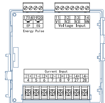
(A2)电压电流信号输入
