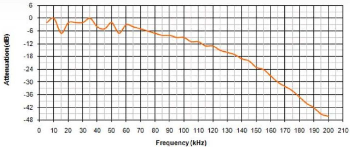
内置扬声器的频率响应
