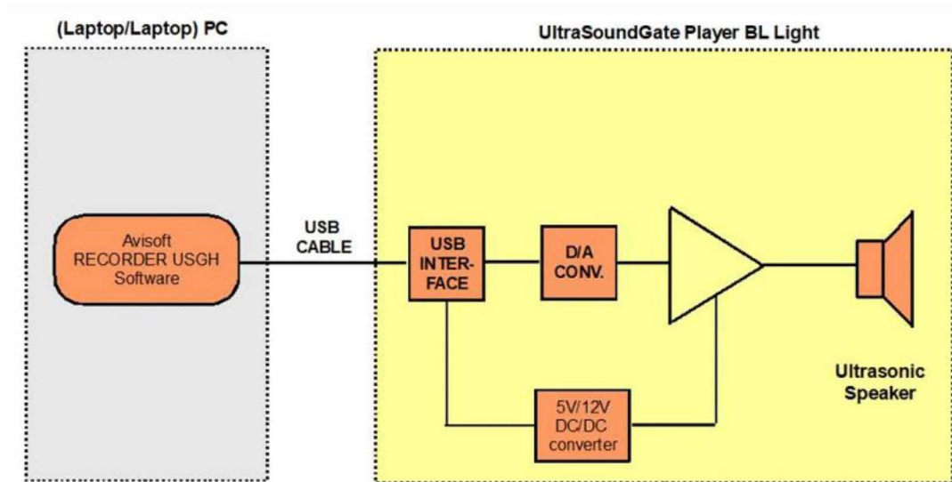
UltraSoundGate Player BL Light 的功能原理
