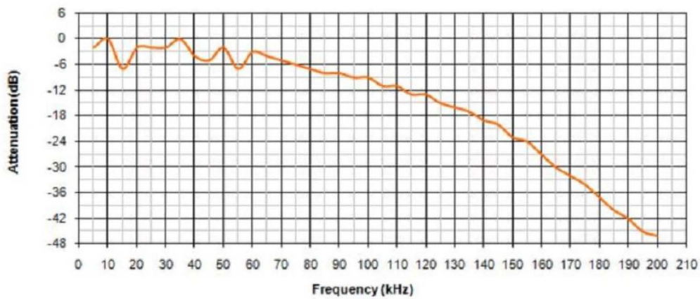
内置扬声器的频率响应
