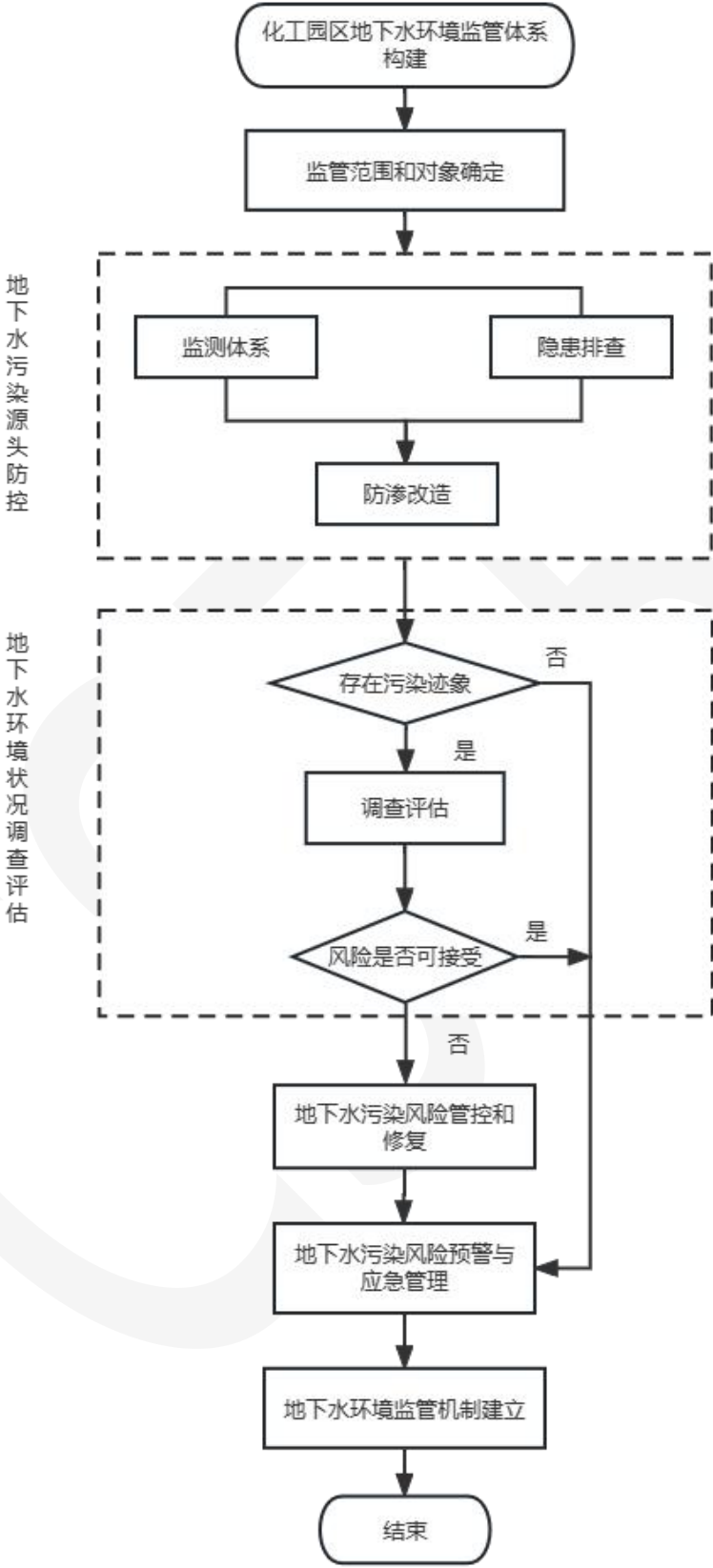
图 1 工作流程图
