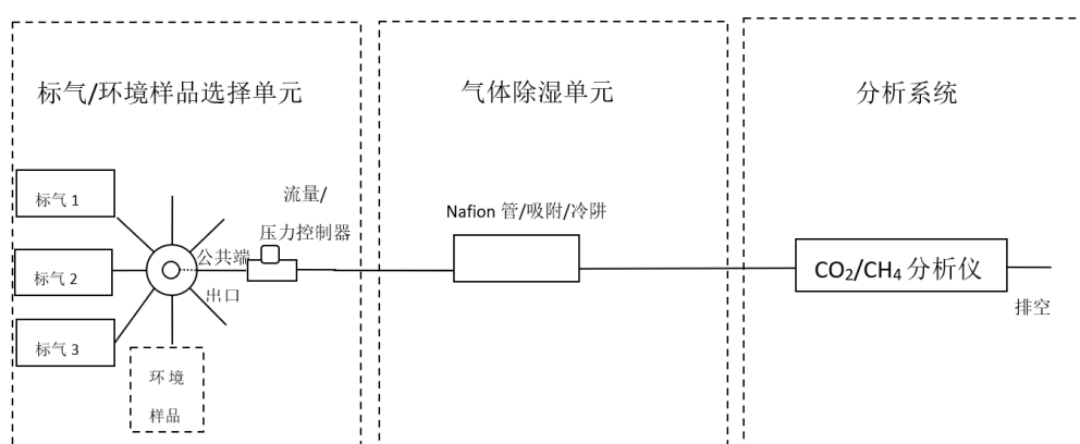
图 1 监测系统示意图
