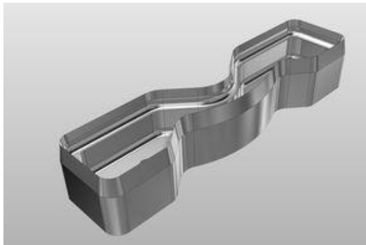
可替换的 DIN ISO 34-1 C 新月型裁切刀片（不带切口）
