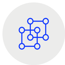
催化剂研究
