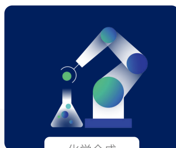
化学合成
