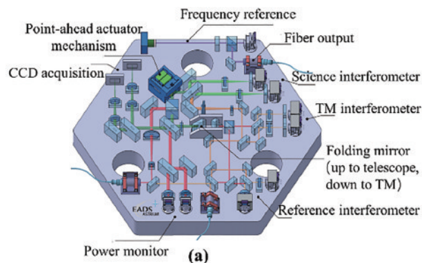
图 13 LISA 光学干涉平台。(a) 2006 [39] ; (b) 2009 [40]
