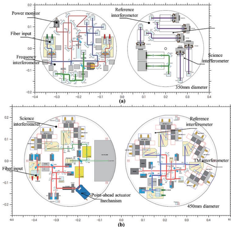
图 17 LISA 光学干涉平台。(a) 2017 [3] ；(b) 2022 [47]
