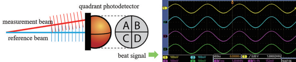
图 7 差分波前传感和四通道拍频信号波形示意图 [25]
