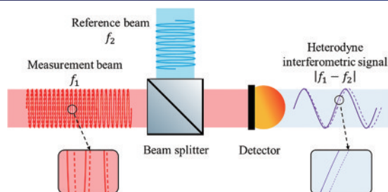
图 5 激光外差干涉原理示意图 [12]
