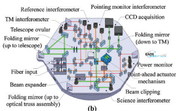
图 13 LISA 光学干涉平台。(a) 2006 [39] ; (b) 2009 [40]
