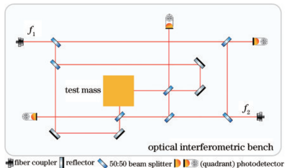
图 22 测试质量五自由度激光外差干涉光路 [57]
