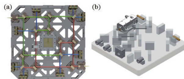
图 23 我国空间引力波探测技术验证卫星激光干涉平台。
