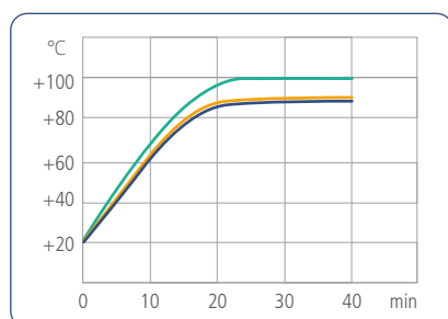
WH280-H 加热曲线
