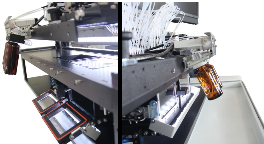
新型 Dx Oligo 192 合成仪
