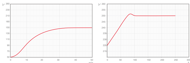
WH200D-2K 使用 1000mL 高温油从 50°C 至 150°C 加热曲线 WH200D-2K 板面温度稳定性 (250°C 数据) (外接 PT100 温度传感器控制)
