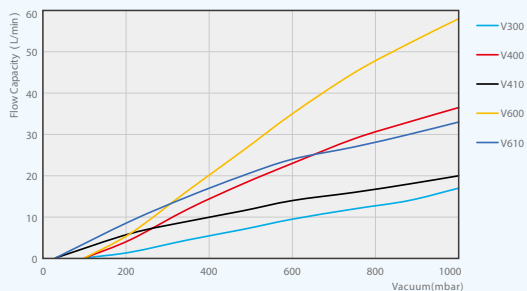
无油真空泵流量曲线图
