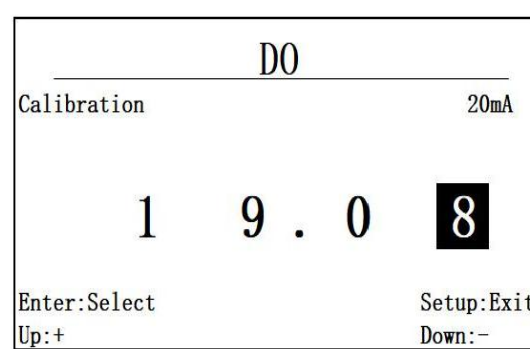
图 6.5 20mA 校准输入 19.08
