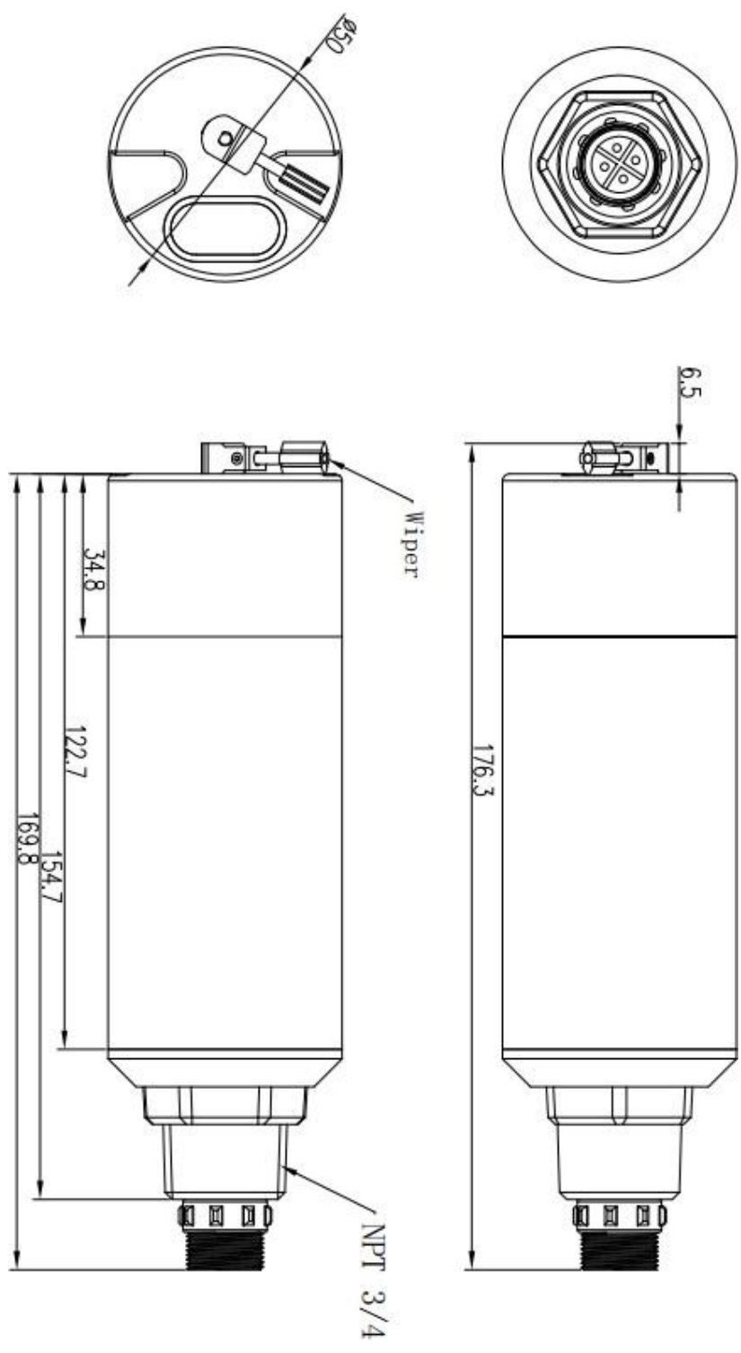
图 1-2 结构图
