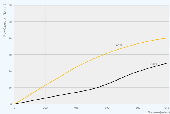
A 泵流量 - 真空曲线图
