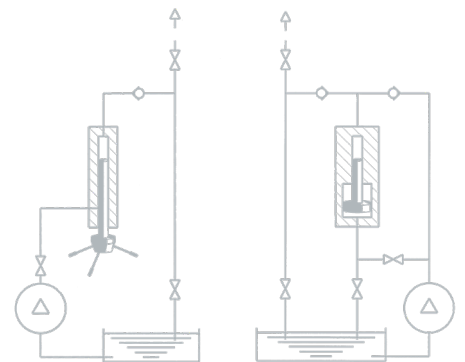
带手泵的台式灭菌系统的流程图
