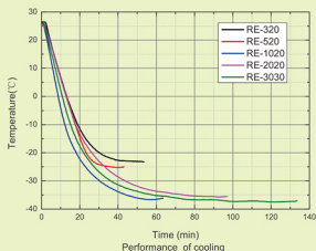
RE 系列 - 冷却曲线 (冷却介质: 乙醇) (制冷效率高)
