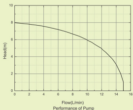
RE-520 / 1020 / 2020 / 3030 磁力泵特性曲线 (高性能磁力泵)
