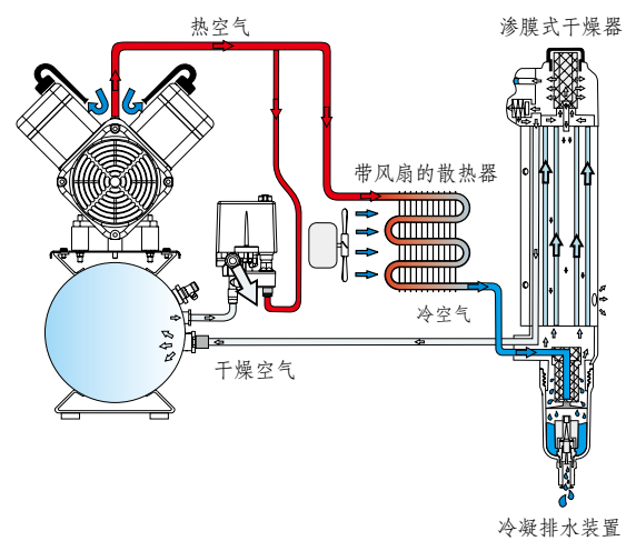
带干燥器的压缩站机能
