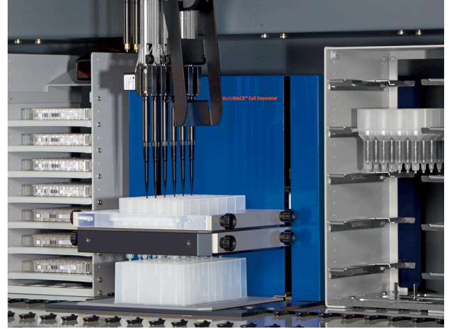
图 3: MultiMACS Cell24 Separator Plus 与自动化液流工作站无缝整合，实现无人看守的全自动细胞分选。
