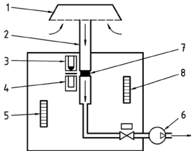
1-切割器；2-进样管；3- \beta 射线放射源；4- \beta 射线检测器；5-空白滤膜；6-泵；7-采样过程中的滤膜；8-采样后滤膜。
