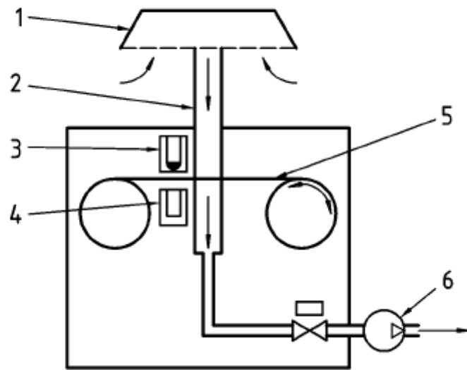
1-切割器；2-进样管；3- \beta 射线放射源；4- \beta 射线检测器；5-滤带；6-泵。
