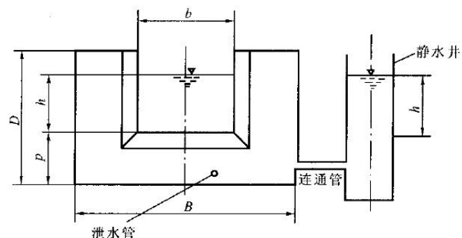
图 D.5 矩形薄壁堰构造示意图
