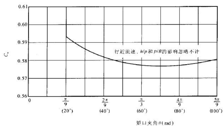
图 D.8 流量系数 C_e 和缺口夹角 \alpha 的关系曲线图
