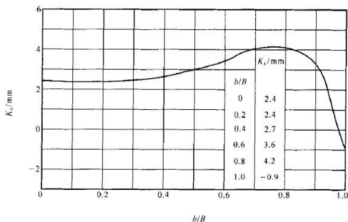
图 D.11 K_e 与 b/B 的关系曲线图
