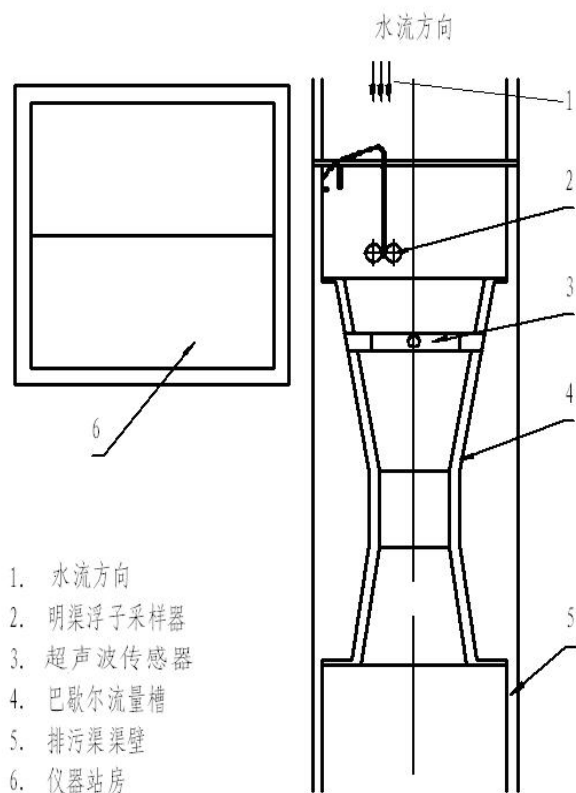
图D. 2 巴歇尔槽现场安装平面示意图
