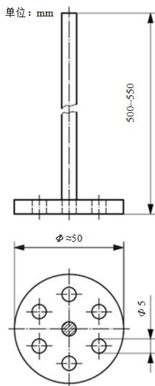
图 2 搅拌器
