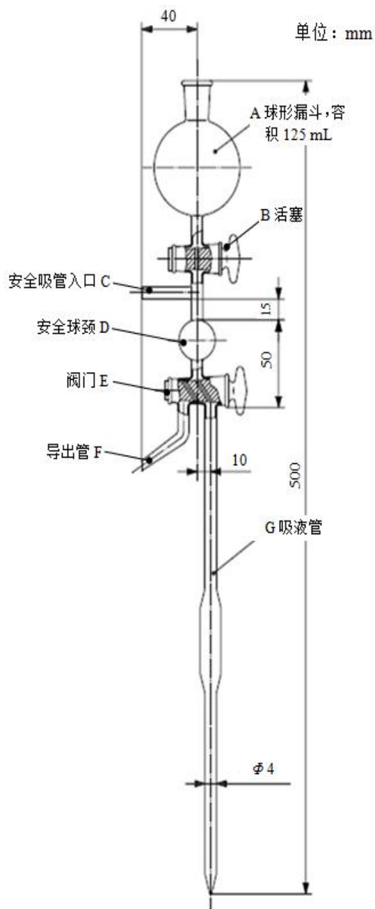
图 1 吸液管
