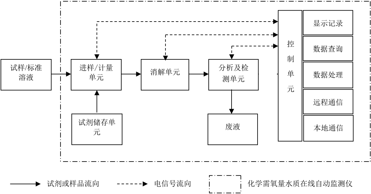
图 1 化学需氧量（COD Cr ）水质在线自动监测仪的基本结构组成图
