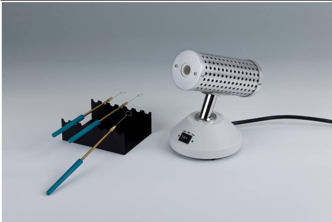
红外接种环灭菌器——JMH3000A
