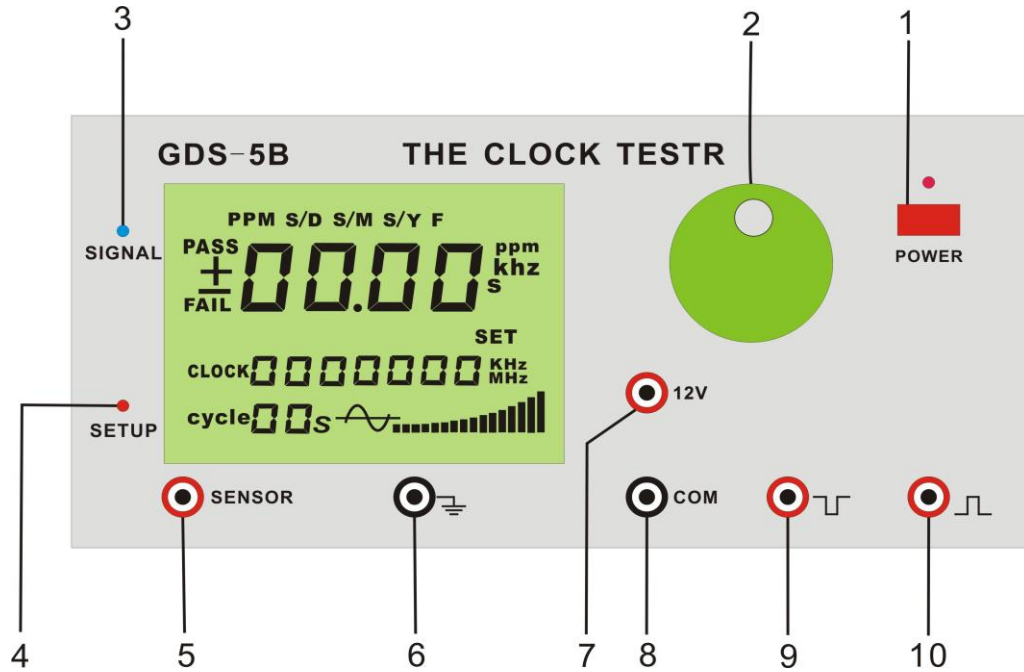
图 2. GDS-5B 时钟测试仪面板（正面）
