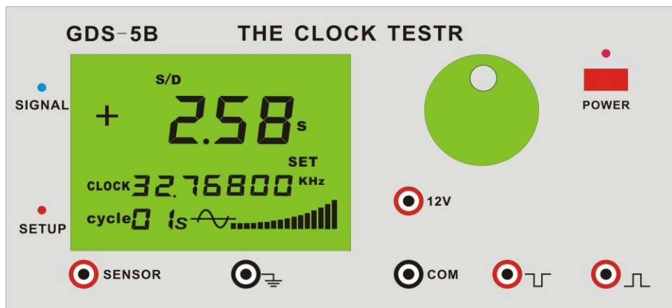
图 6. 显示测量结果界面
