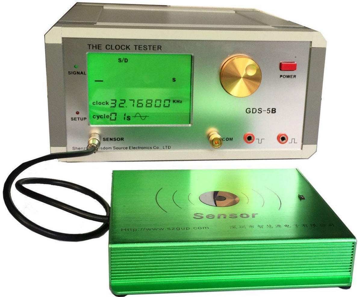
图 1. GDS-5B 时钟测试仪
