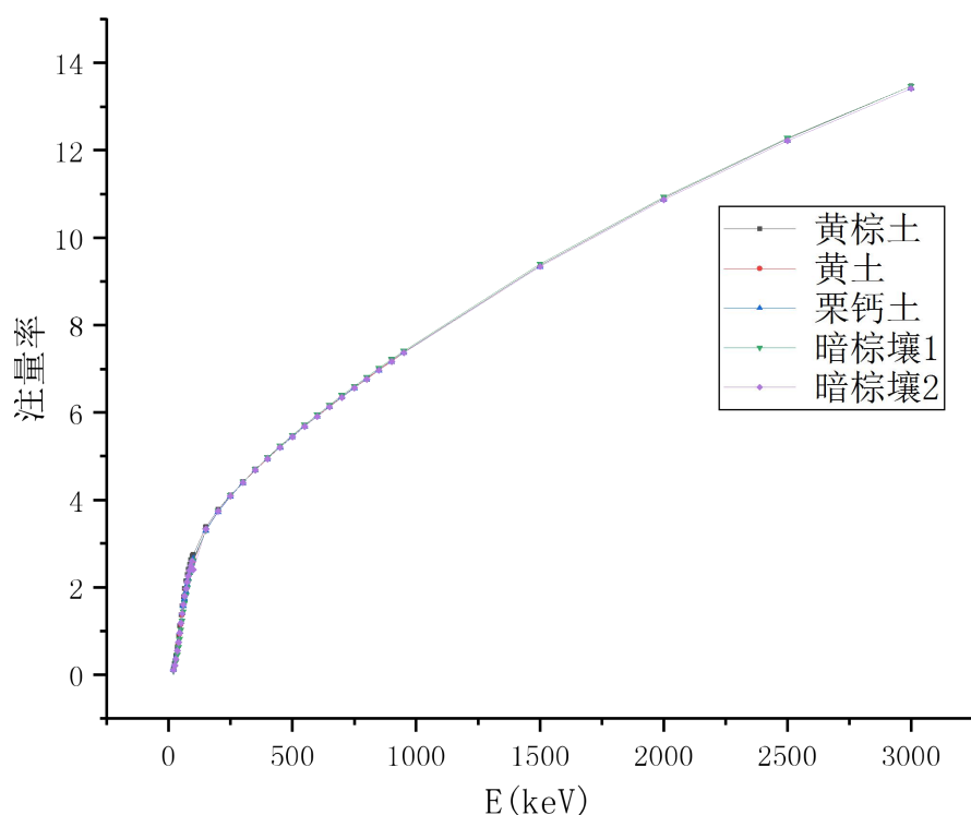
图 3 不同土壤组分在地表 1m 处产生的 \gamma 射线注量率
