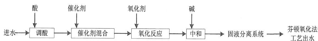
图 1 芬顿氧化法废水处理工程工艺流程图
