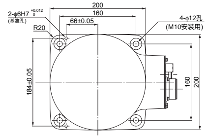
底座安装面 (从上面看)
