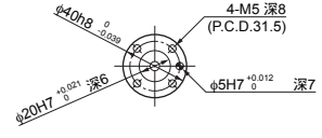
底座安装面 (从上面看)
