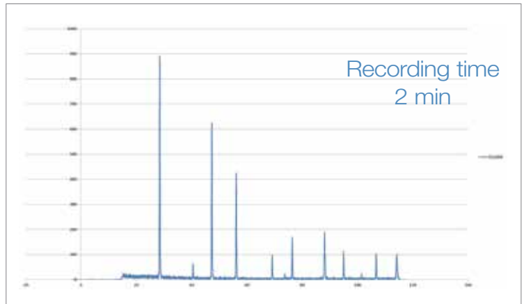
ARL EQUINOX 1000在反射模式下测试Si粉末的数据
