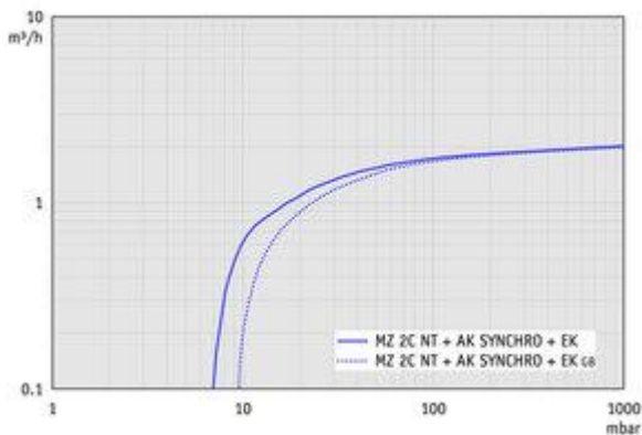
MZ 2C NT +AK SYNCHRO+EK - 60 Hz 下的抽速曲线
