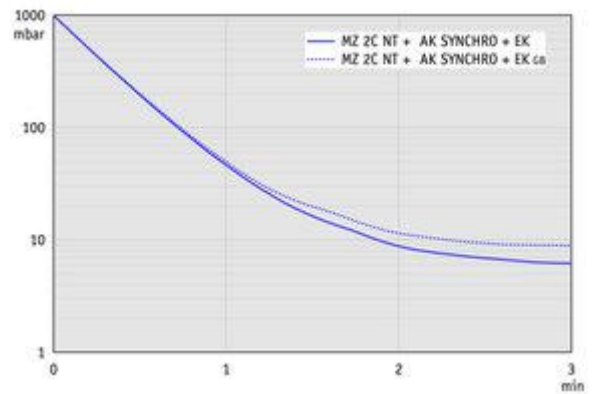
MZ 2C NT +AK SYNCHRO+EK - 60 Hz 下的抽气曲线 (10 升容积)
