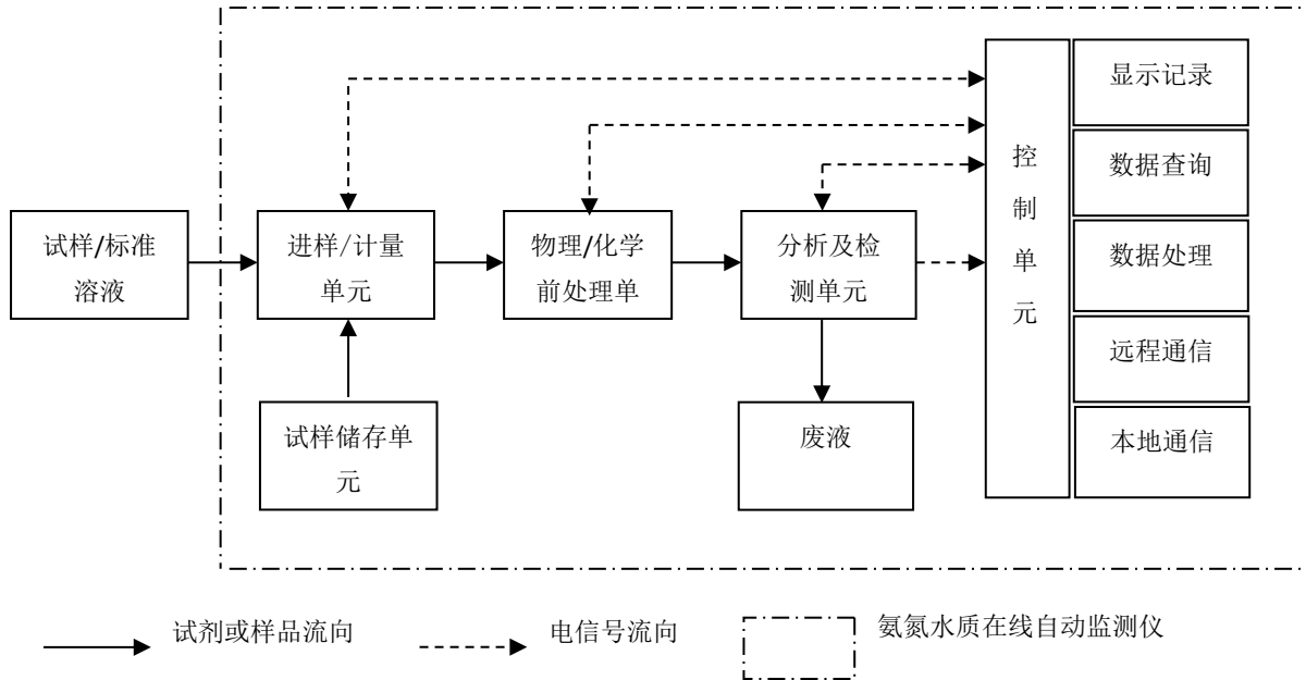
图 1 氨氮水质在线自动监测仪的基本结构组成图
