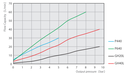
压力泵输出压力与流量曲线
