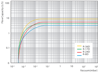
抽气速率曲线
