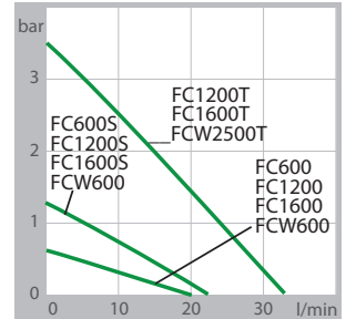
泵功率示意图 使用浴液: 水
