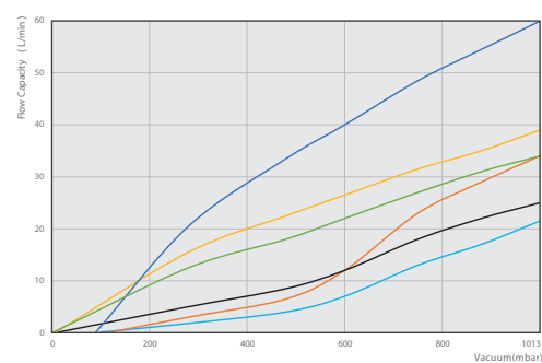
防腐蚀隔膜真空泵流量曲线图
