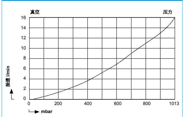
流量曲线
