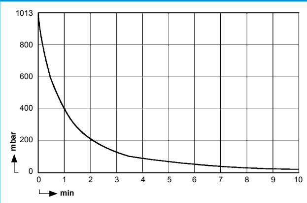
连10升的容器下泵抽真空的时间曲线
