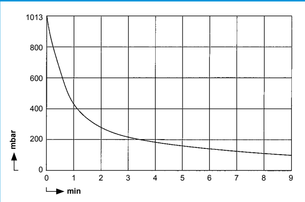
连5升的容器下泵抽真空的时间曲线
