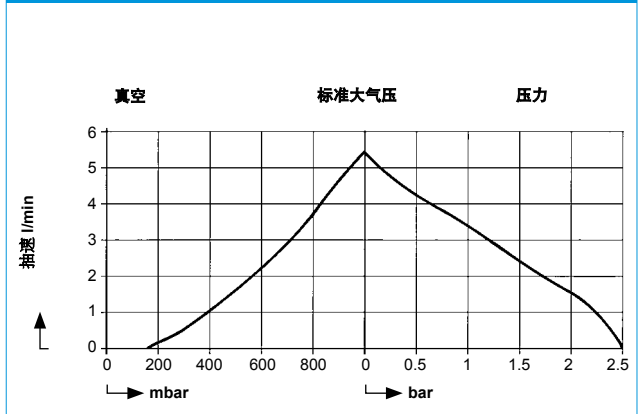
流量曲线
