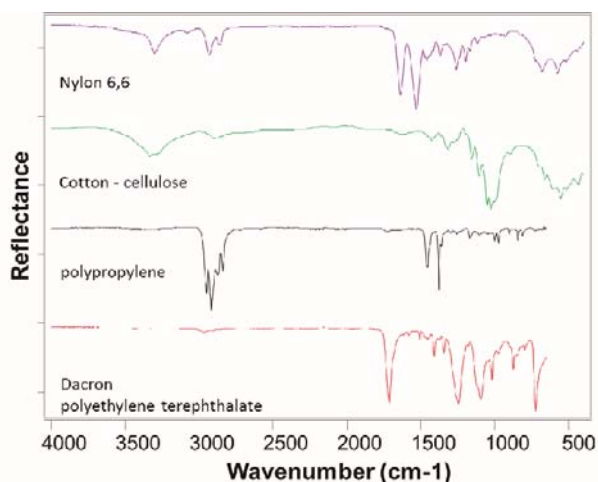
下图：纤维在ATR下得到的红外光谱图
