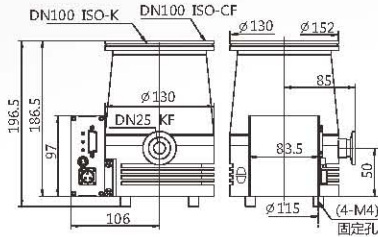
FF-100/150外形尺寸图
