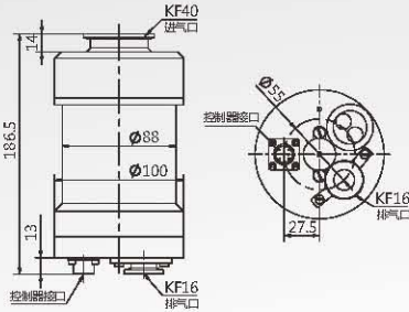
FF-40/25外形尺寸图
