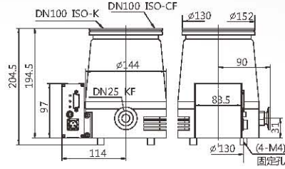
FF-100/300外形尺寸图
