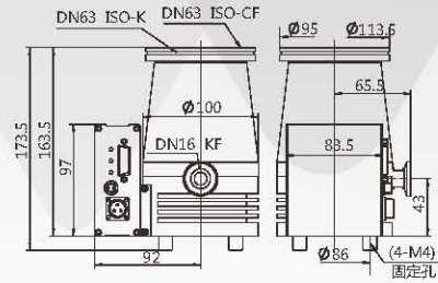
FF-63/80外形尺寸图
