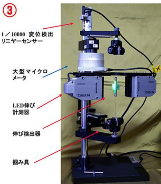
伸び計検出器校正装置
