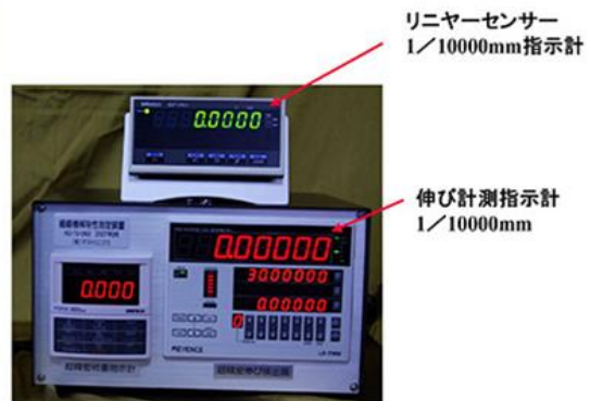
伸び計検出器校正装置
